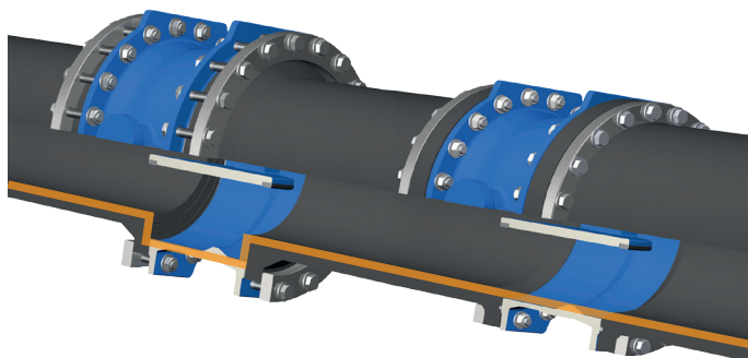
Reducerad fläns (SF)
