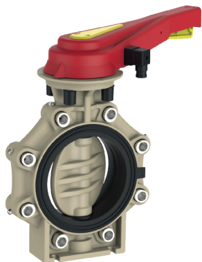
Säkerhetshandtag med induktiv eller mekanisk återkoppling
