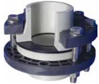
GSTP gummipackning med profil anpassad för plaströrssystem.
