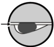
Tätning genom rund tätningsprofil
